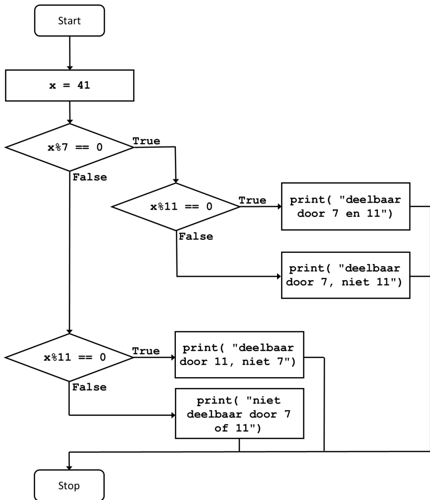
Afb. 6.3: Stroomdiagram dat een geneste conditie weergeeft.
