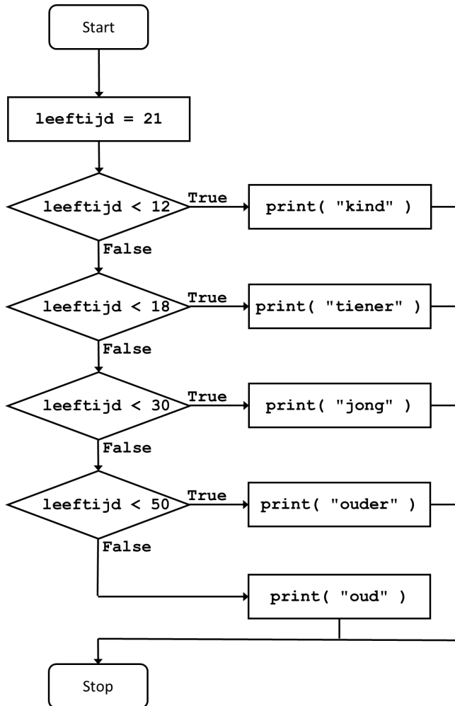
Afb. 6.2: Stroomdiagram dat een meer-weg beslissing weergeeft.
