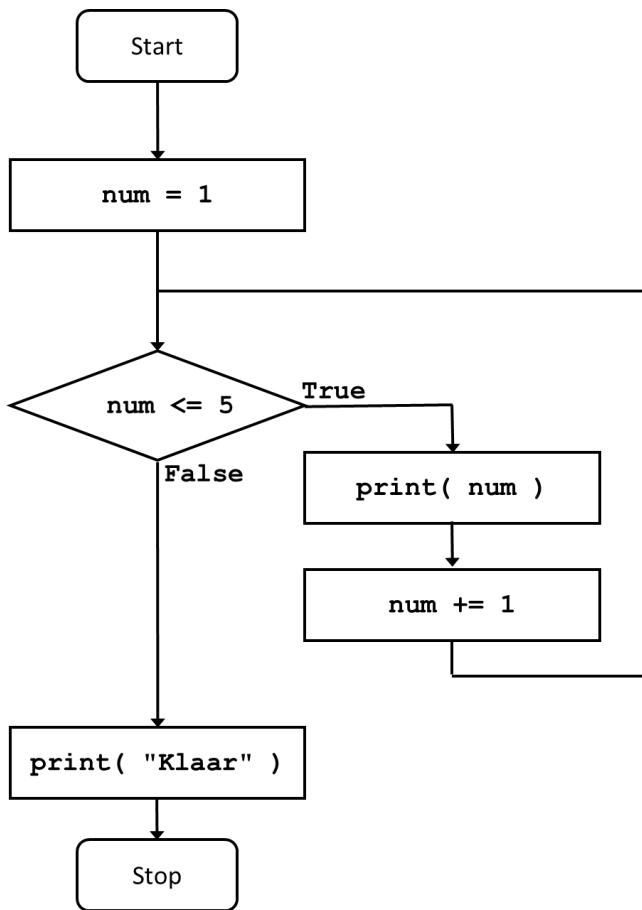
Afb. 7.1: Stroomdiagram dat een while loop weergeeft.
